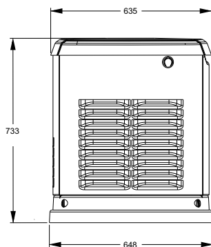
左側面図
